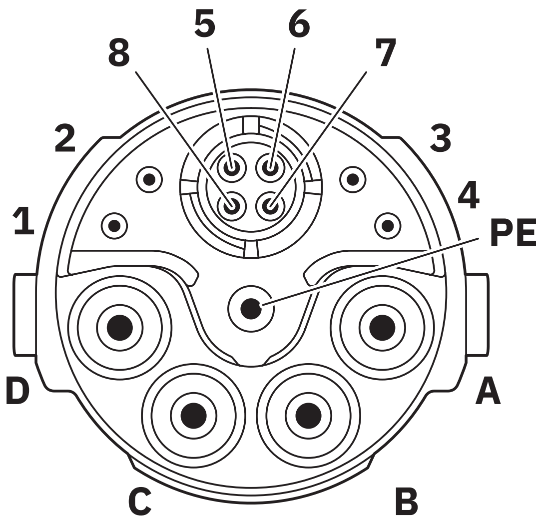
Dessin schématique
