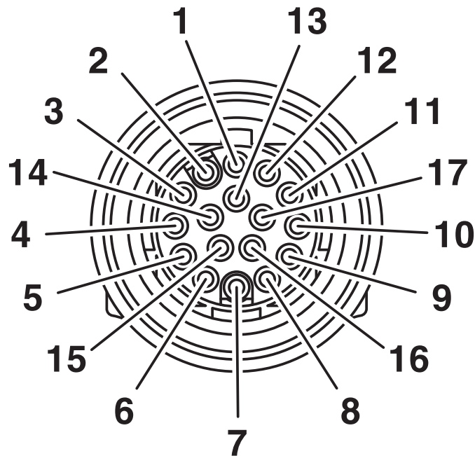
Dessin schématique
