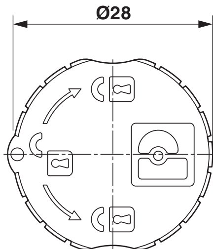
Dessin coté
