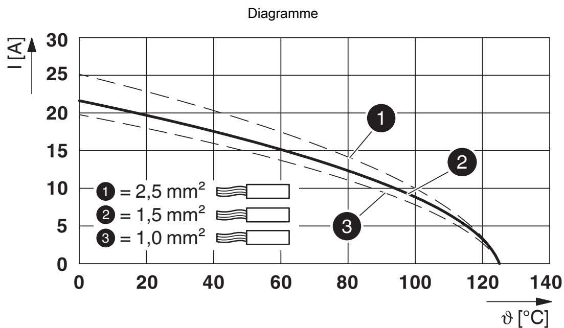
Diagramme de déclassément pour les conducteurs rigides
