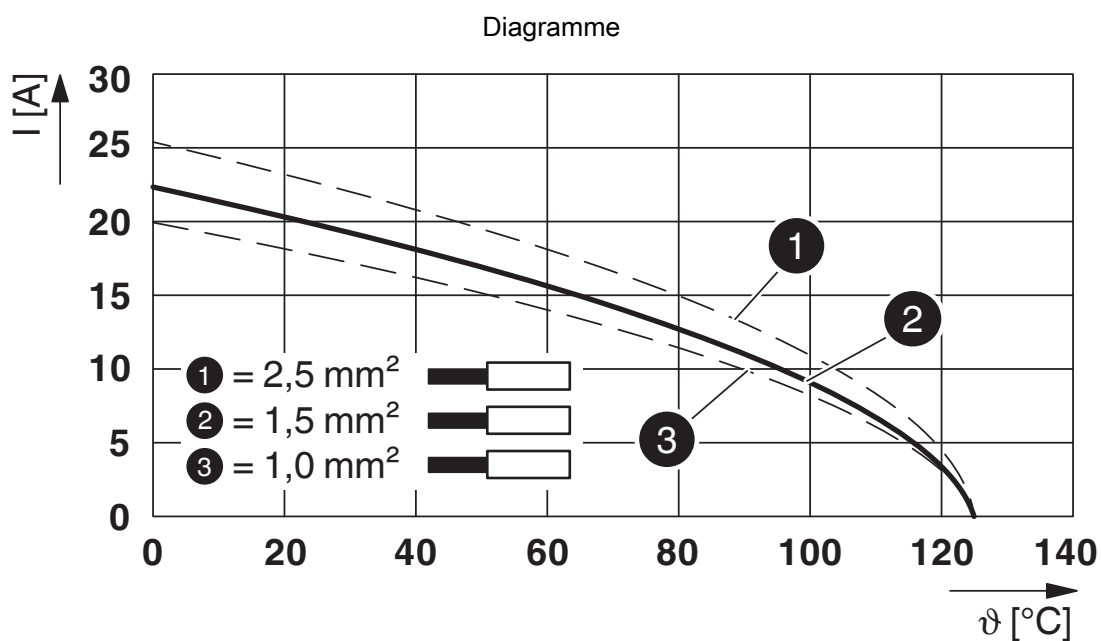
Diagramme de déclassement pour les conducteurs rigides
