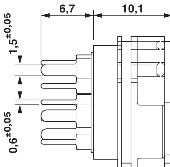
Dessin coté
