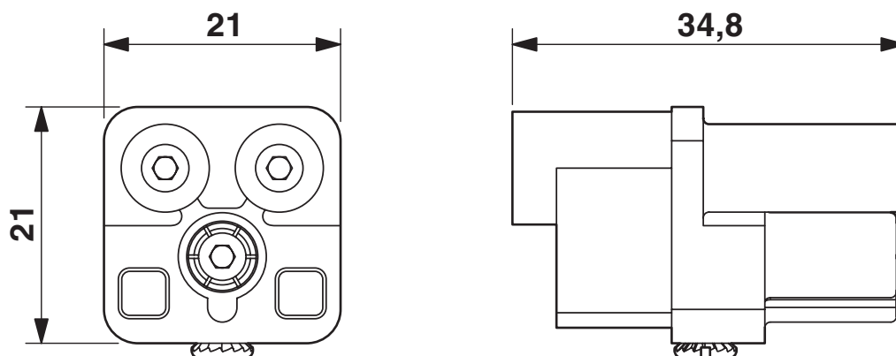
Dessin coté
