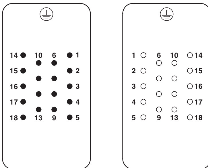
Dessin schématique
