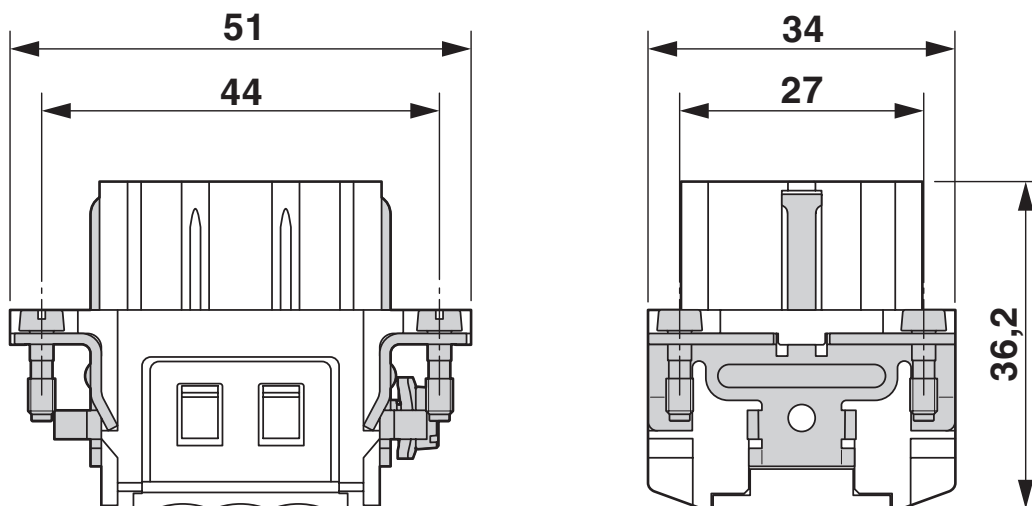
Dessin coté
