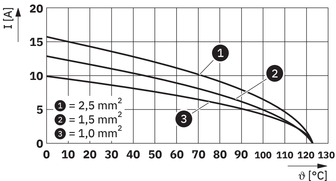
Courbe de derating, contacts roulés
