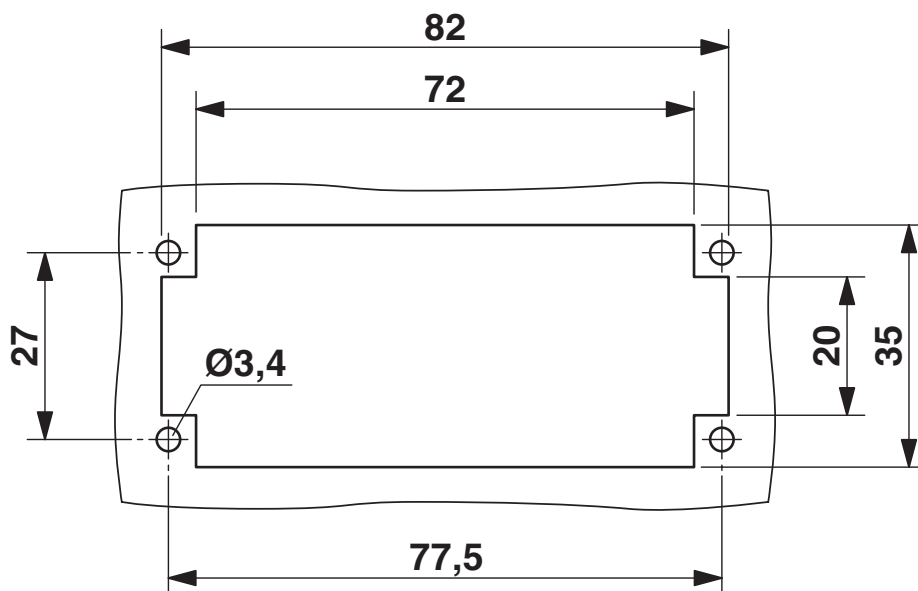
Dessin coté
