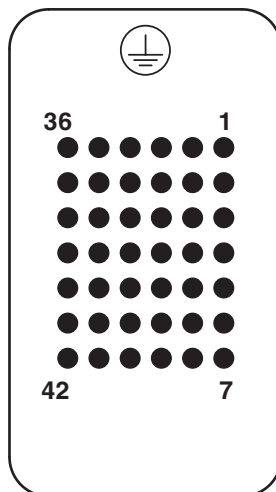
Dessin schématique
