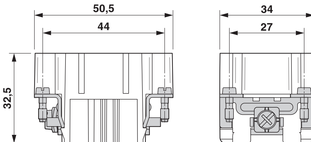
Dessin coté
