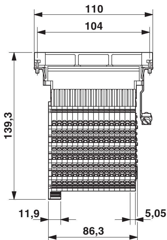
Dessin coté
