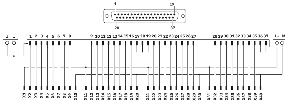
Schéma de connexion
