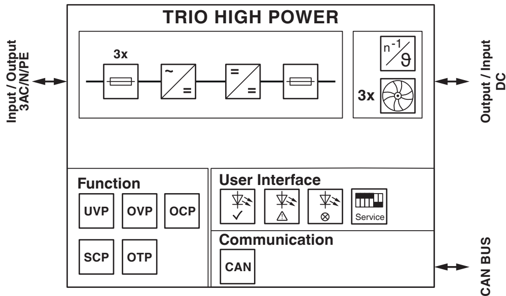
Schéma fonctionnel
