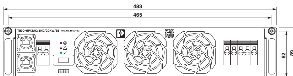
Dessin coté
