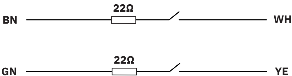
Schéma de connexion
