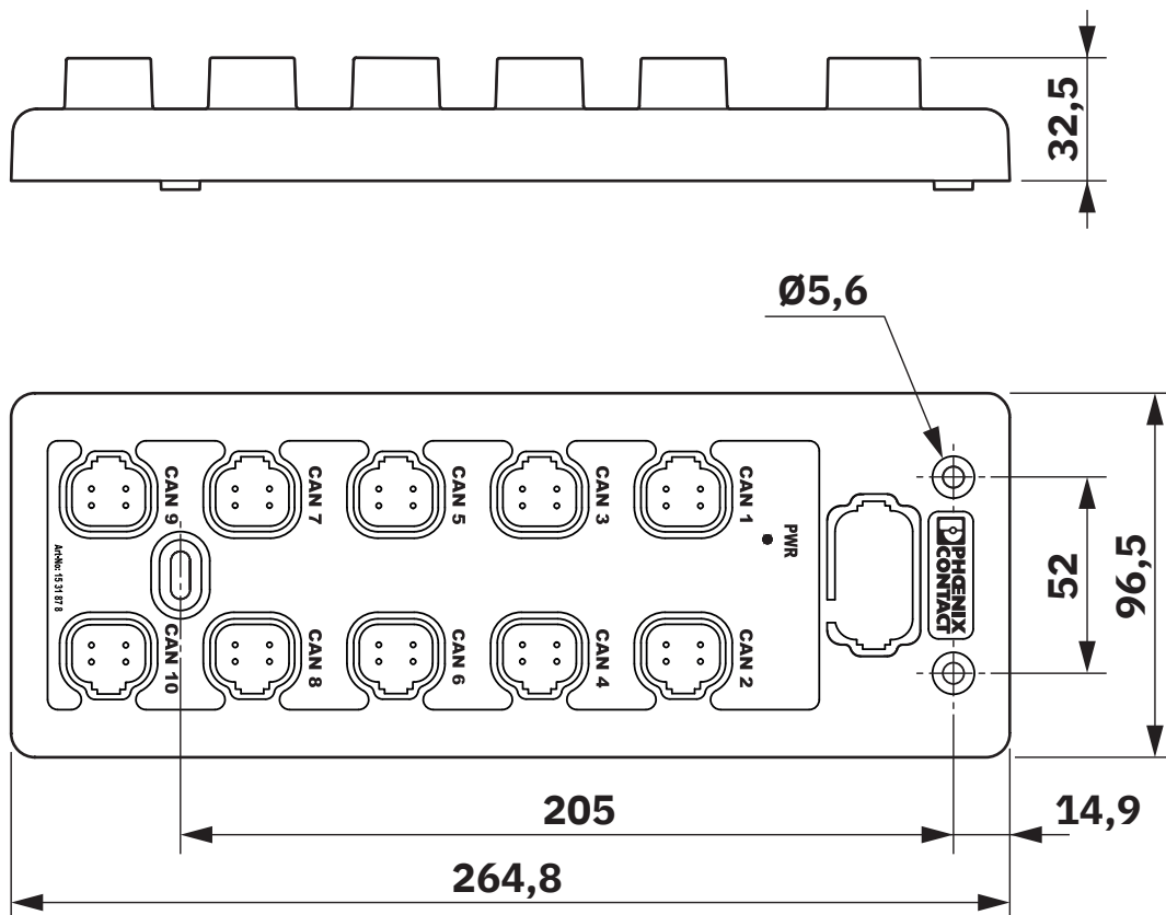
Dessin coté
