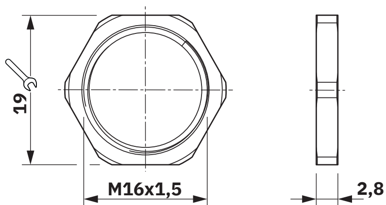
Dessin coté
