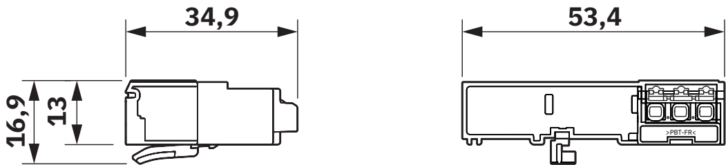
Dessin coté
