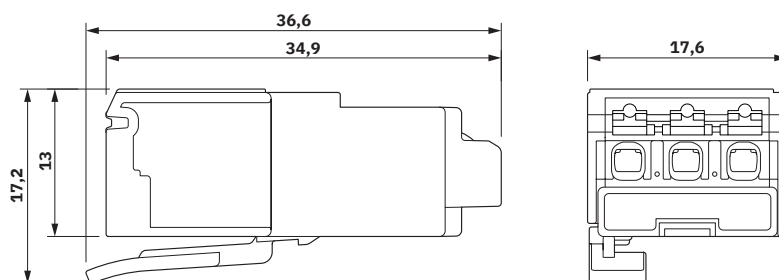
Dessin coté
