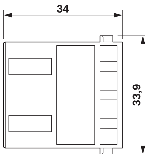
Dessin coté
