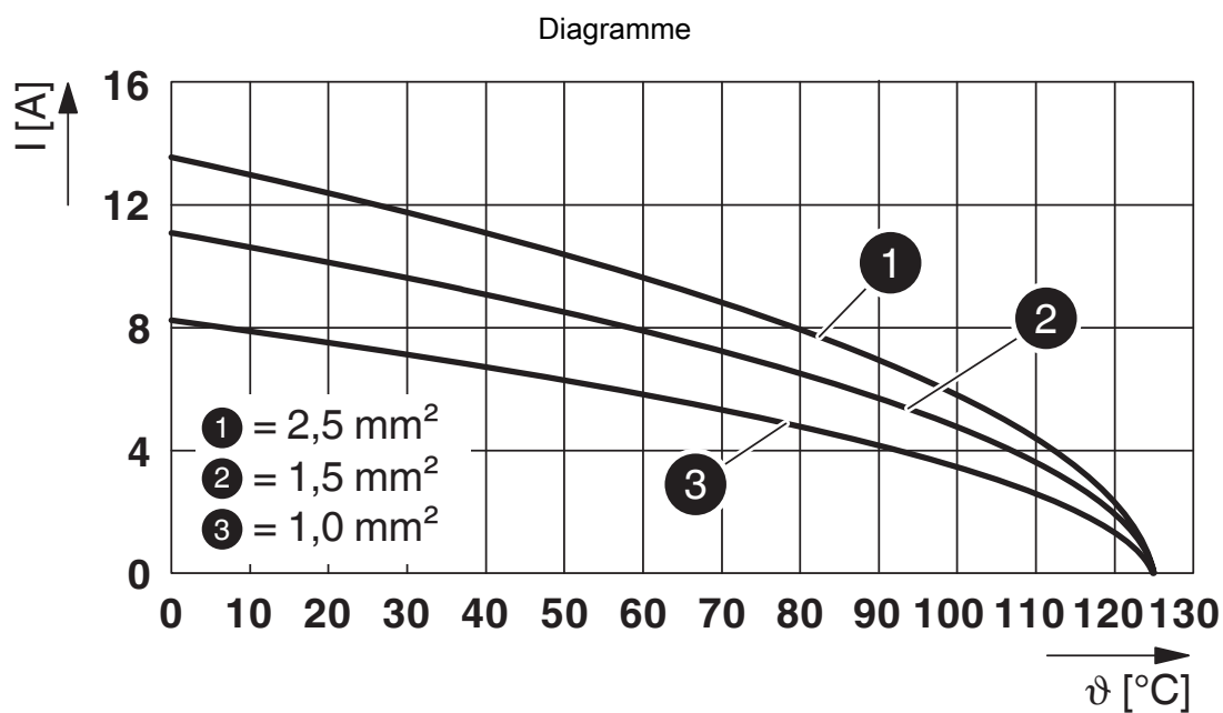
Courbe de derating - contacts tournés
