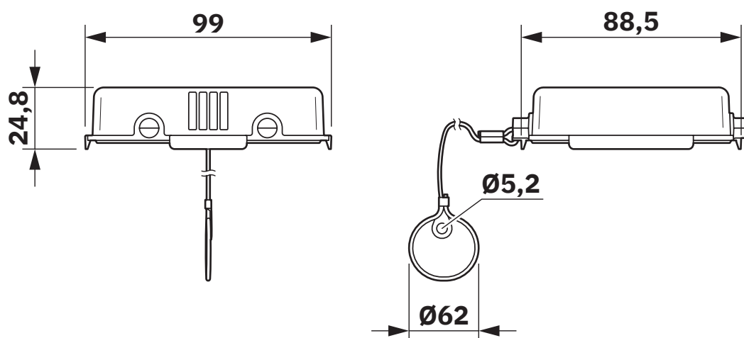
Dessin coté
