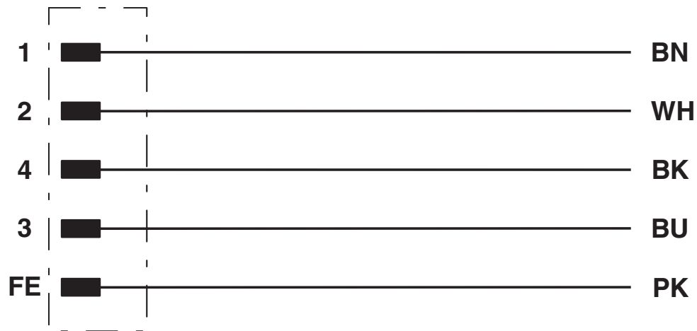
Affectation des contacts du connecteur mâle M12
