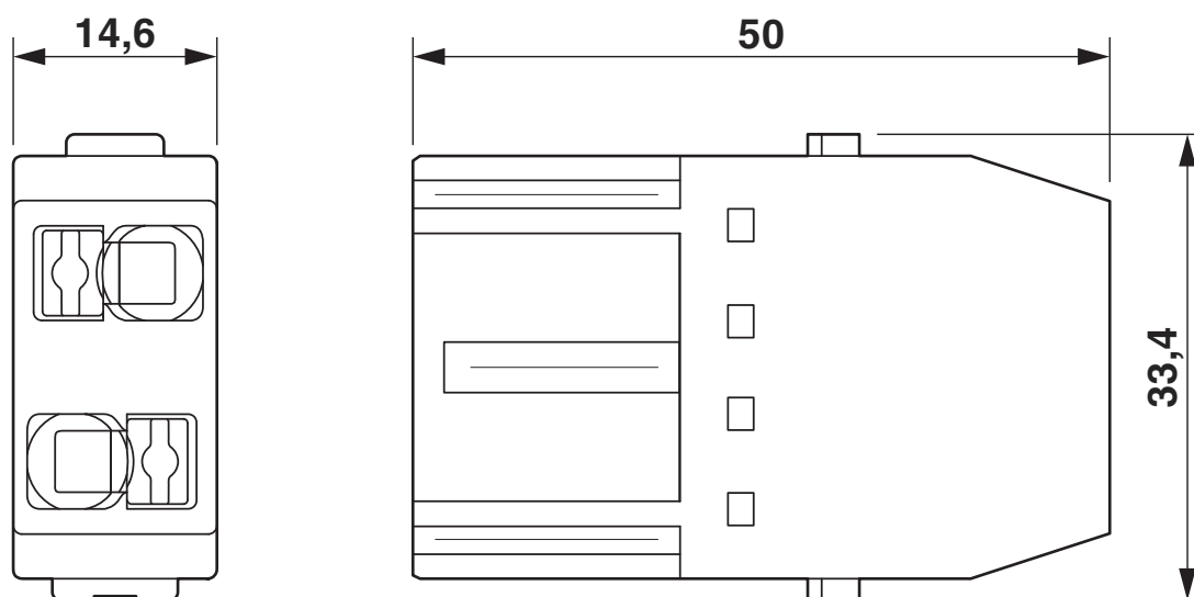
Dessin coté
