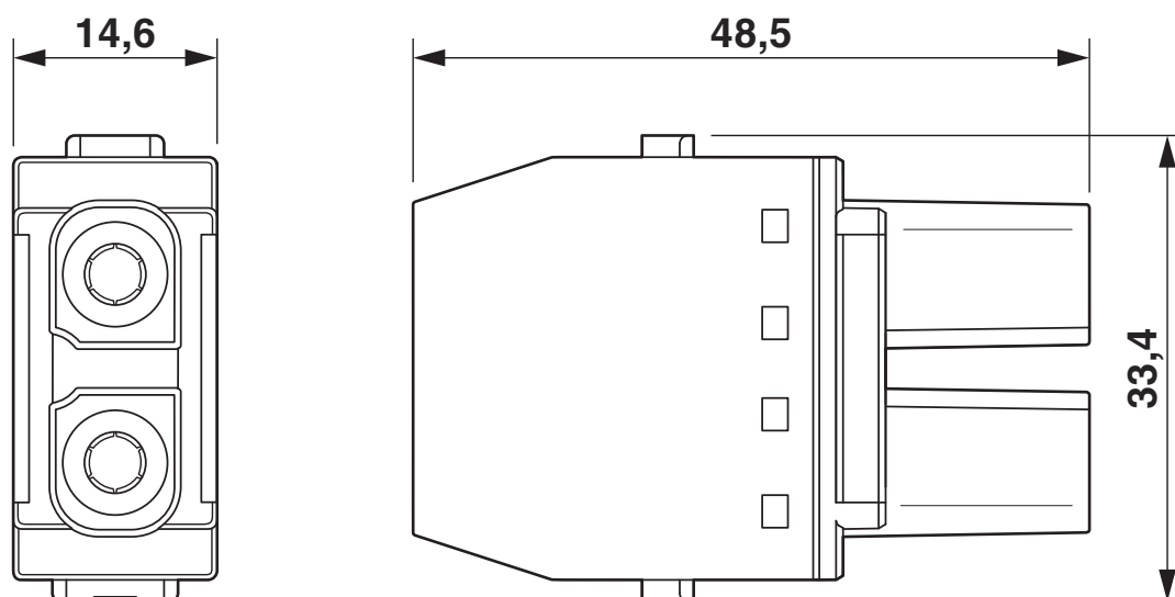
Dessin coté
