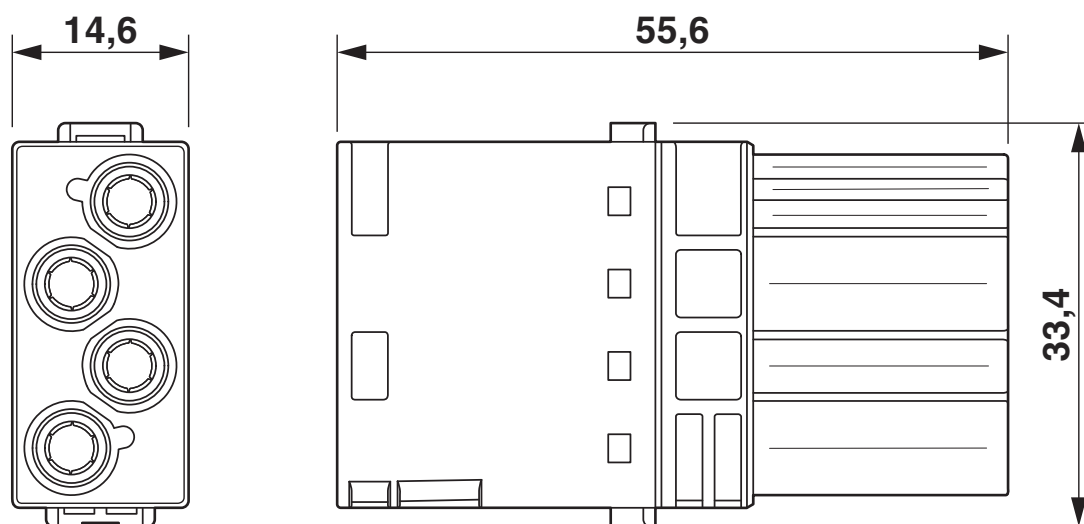
Dessin coté
