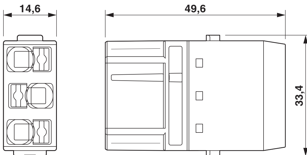
Dessin coté
