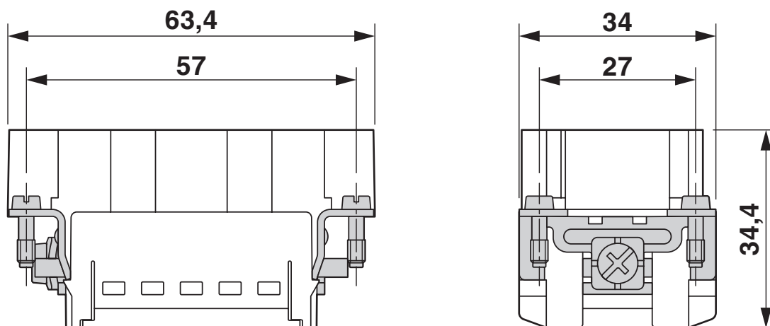
Dessin coté
