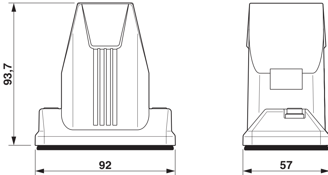
Dessin coté
