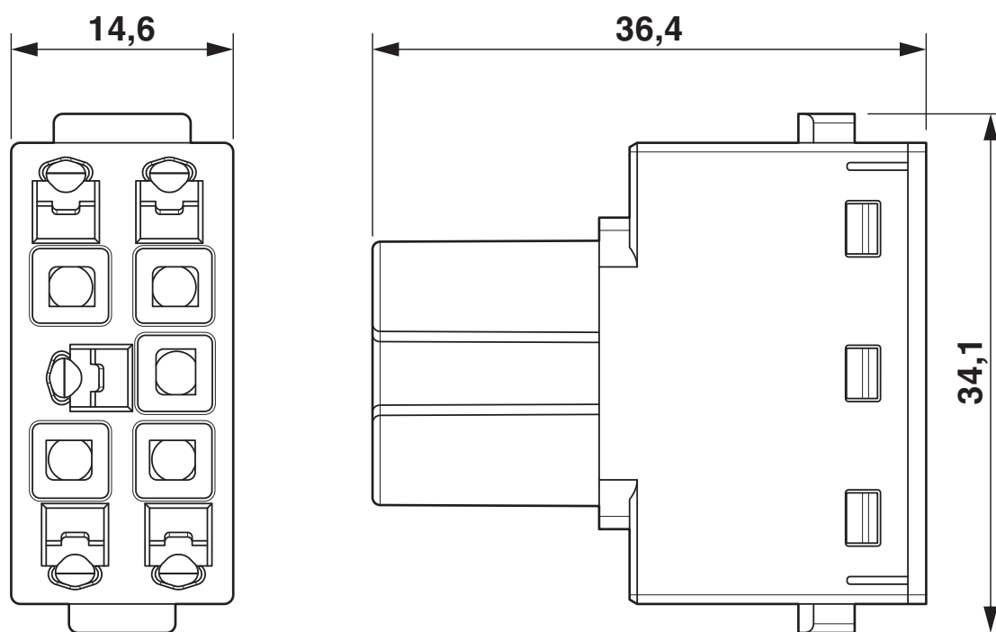
Dessin coté
