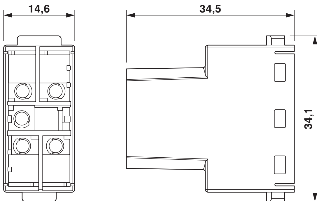
Dessin coté
