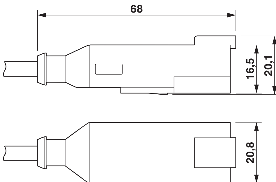
Dessin coté
