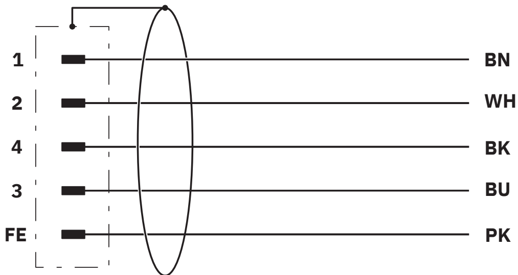
Affectation des contacts du connecteur mâle M12
