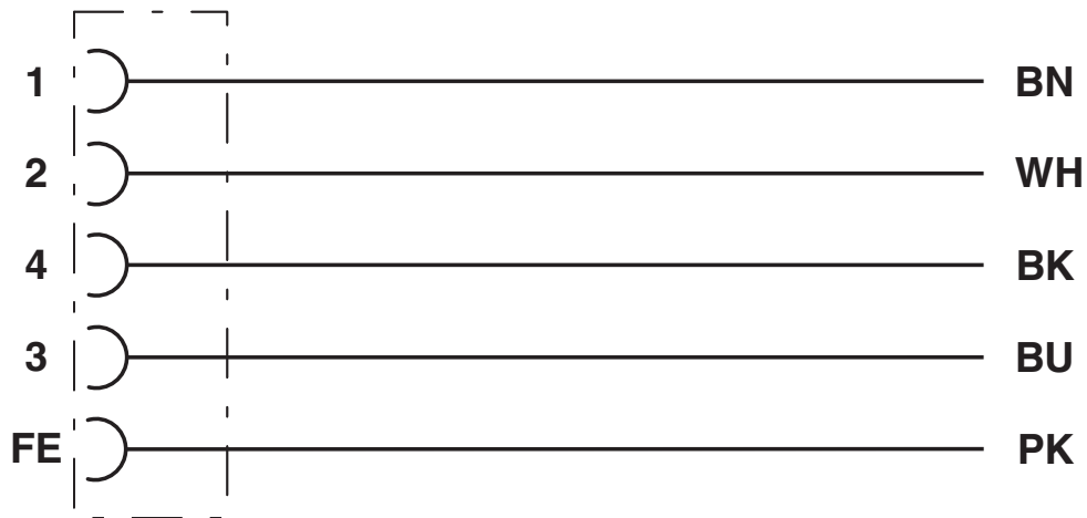
Affectation des contacts du connecteur femelle M12
