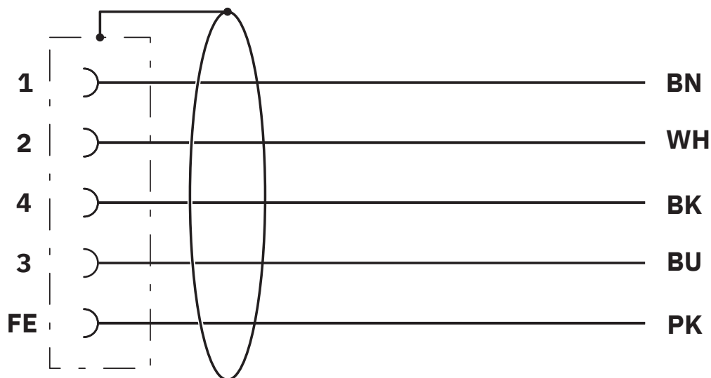
Affectation des contacts du connecteur femelle M12
