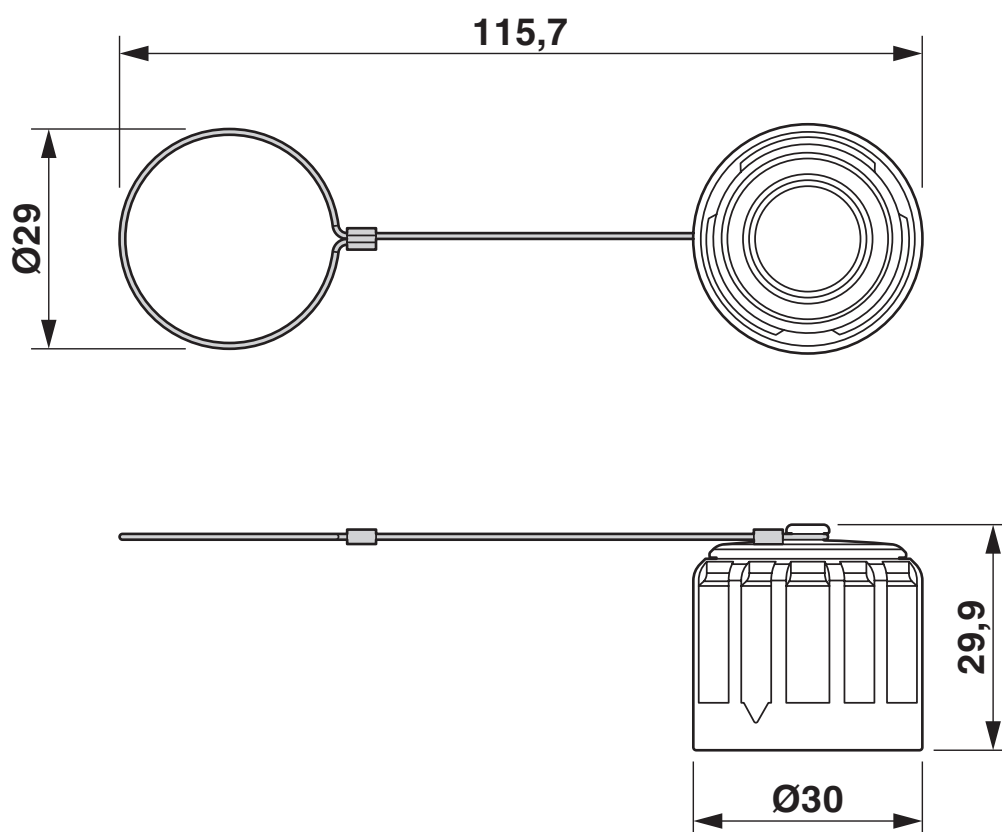
Dessin coté
