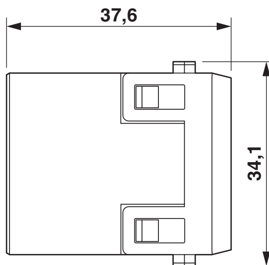
Dessin coté
