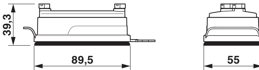
Dessin coté
