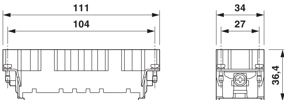
Dessin coté
