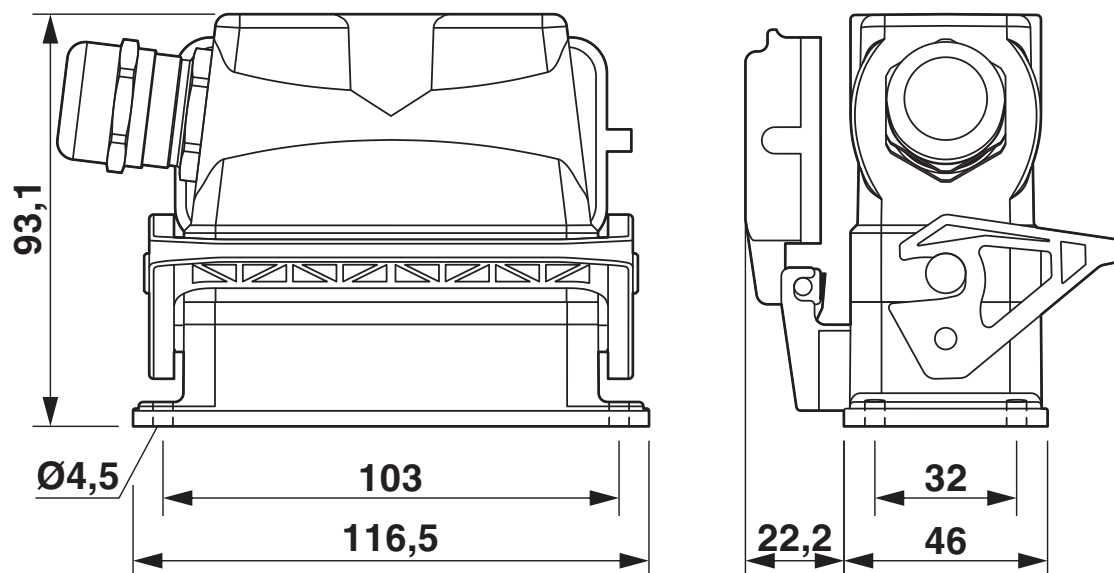
Dessin coté
