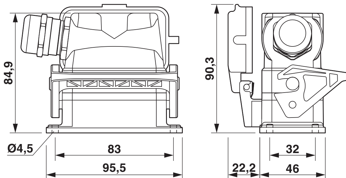
Dessin coté
