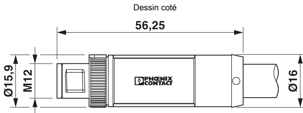
Connecteur mâle M12 x 1, droit
