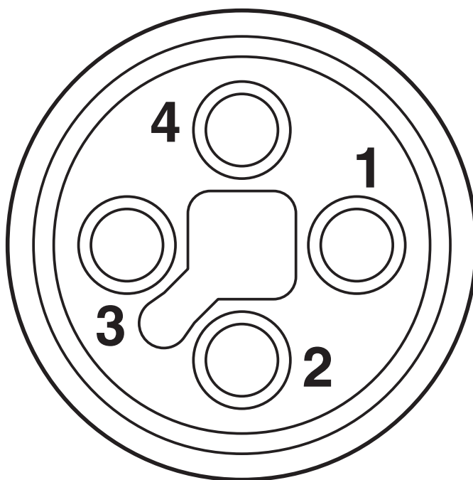
Nombre de pôles M12 femelle, 4 pôles, détrompage T, vue côté femelle
