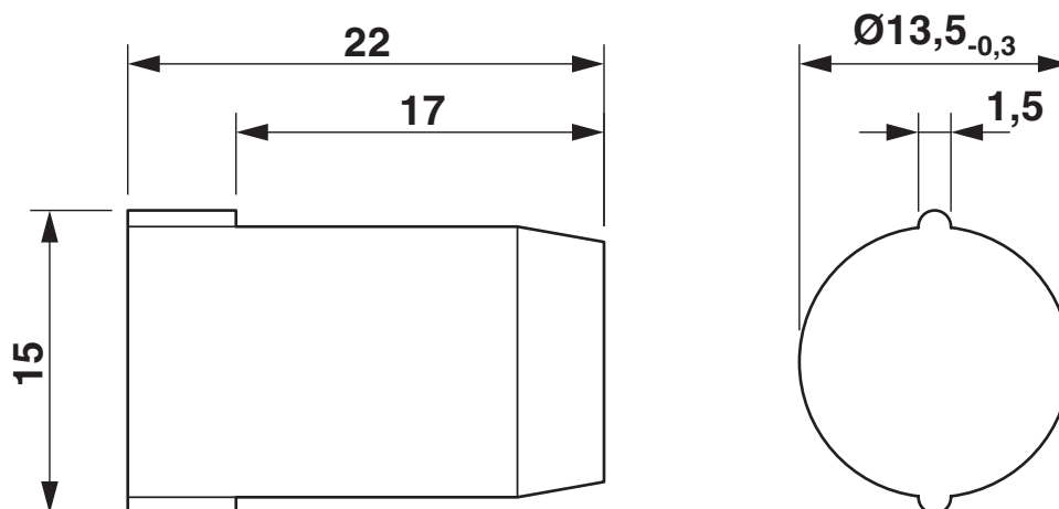
Dessin coté
