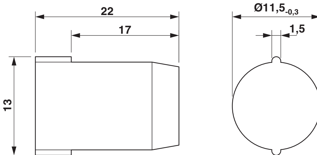
Dessin coté
