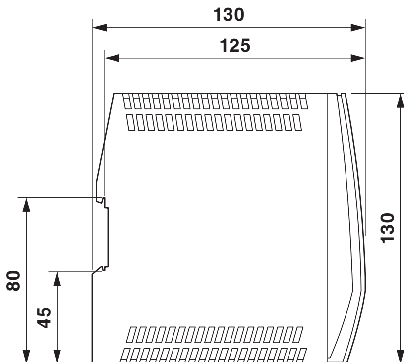
Encombrement de l'appareil (cotes en mm)
