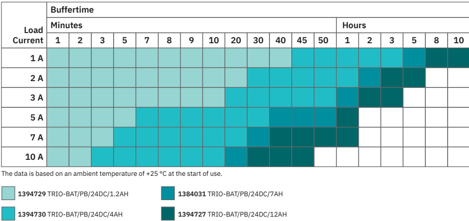
Durées d'autonomie de batterie TRIO pour TRIO3-UPS
