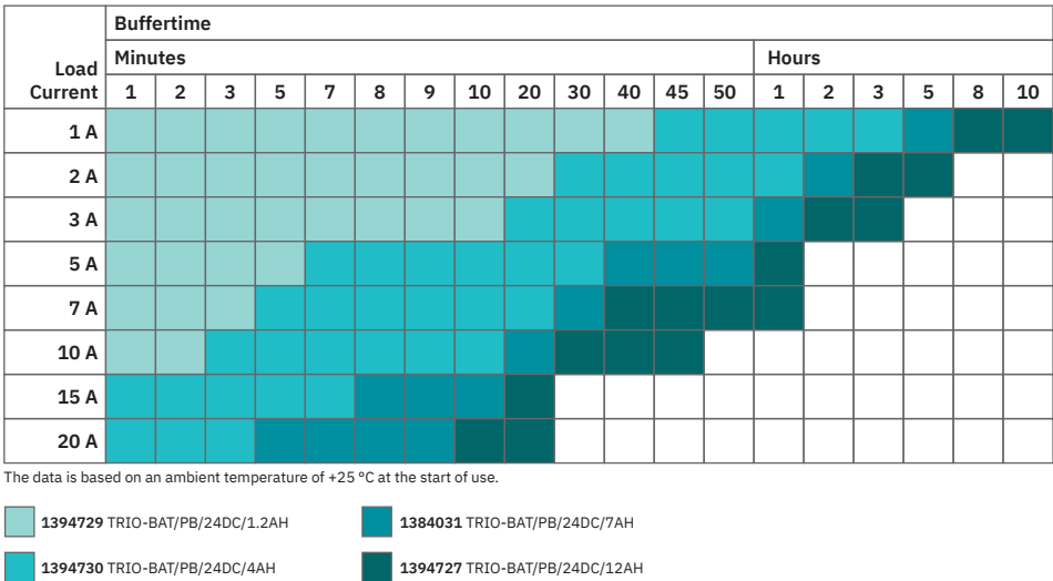
Durées d'autonomie de batterie TRIO pour TRIO-UPS-2G
