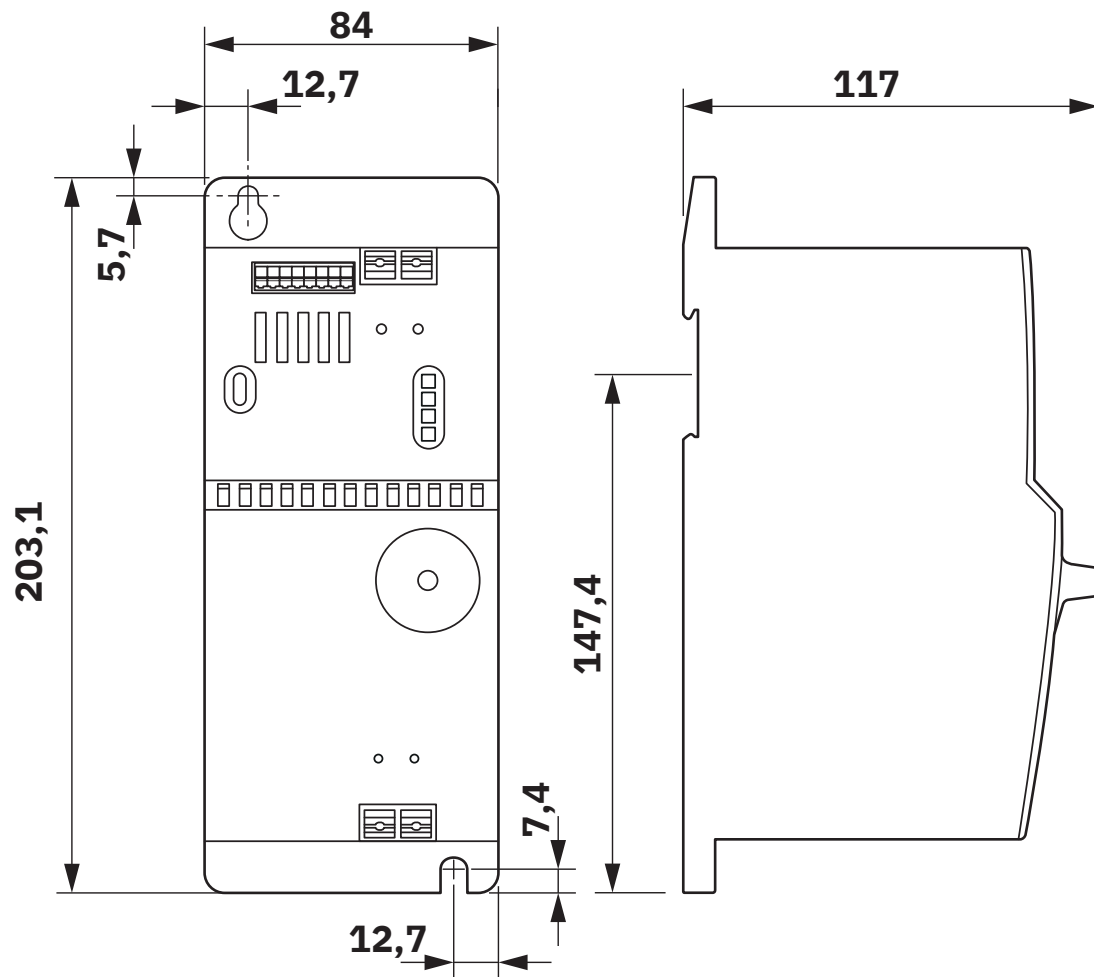
Dessin coté
