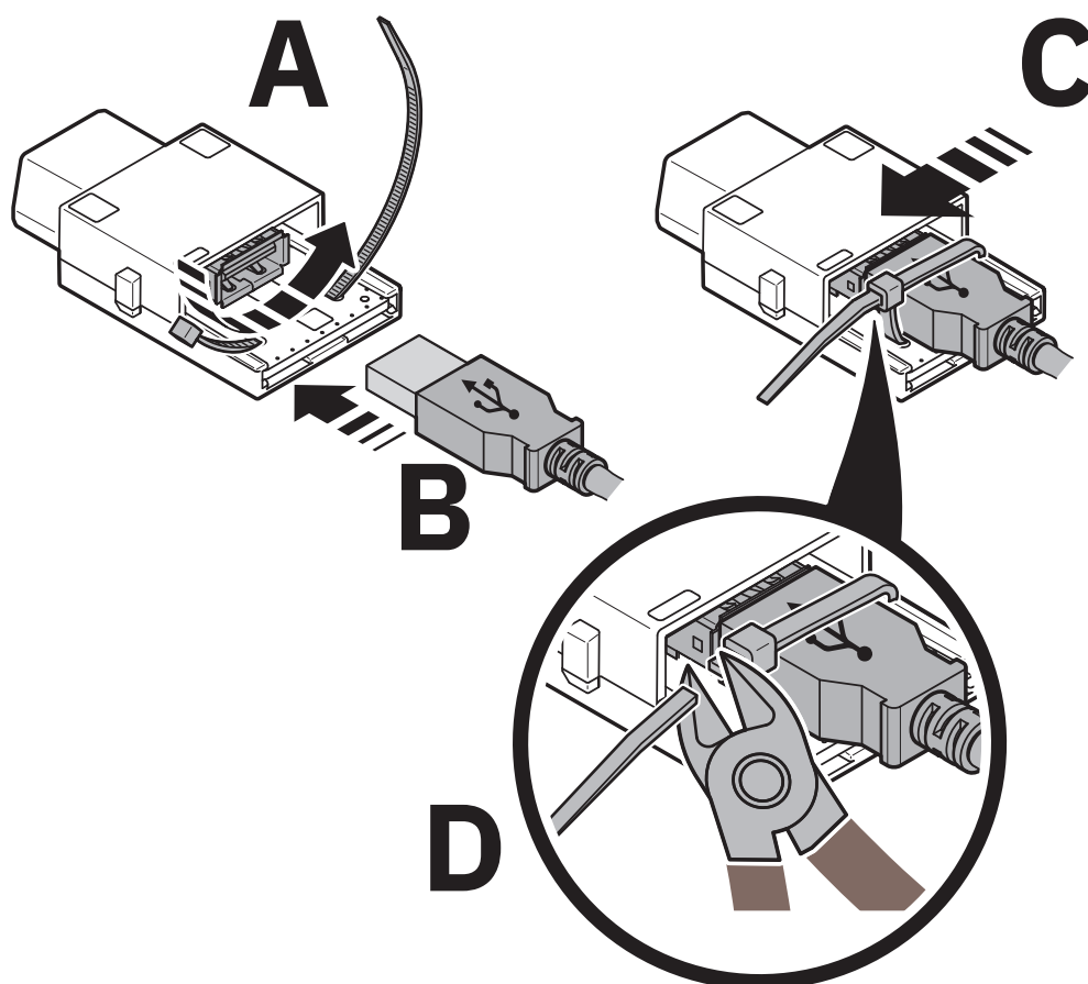
Dessin schématique
